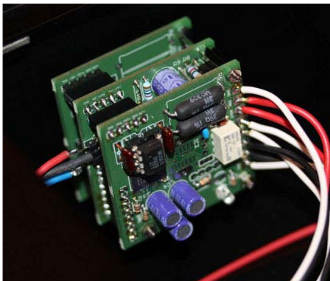
3 枚ボード仕様とした AEDIO EVR-3 回路構成、使用パーツは市販品とまったく同じ (新日本無線株式会社様ご提供)
