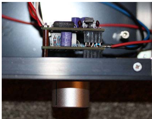
オペアンプを交換するため、電源基板を前に、電子ボリューム基板を後方に配置した EVR-3 (新日本無線株式会社様ご提供)
