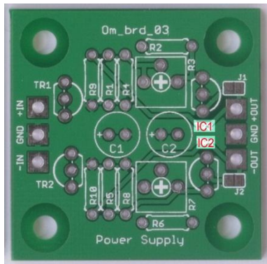
図1 レギュレータ基板
